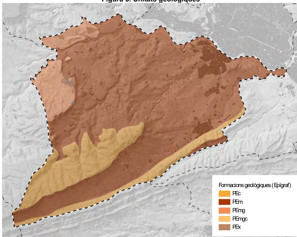
Figura 6. Unitats geològiques
